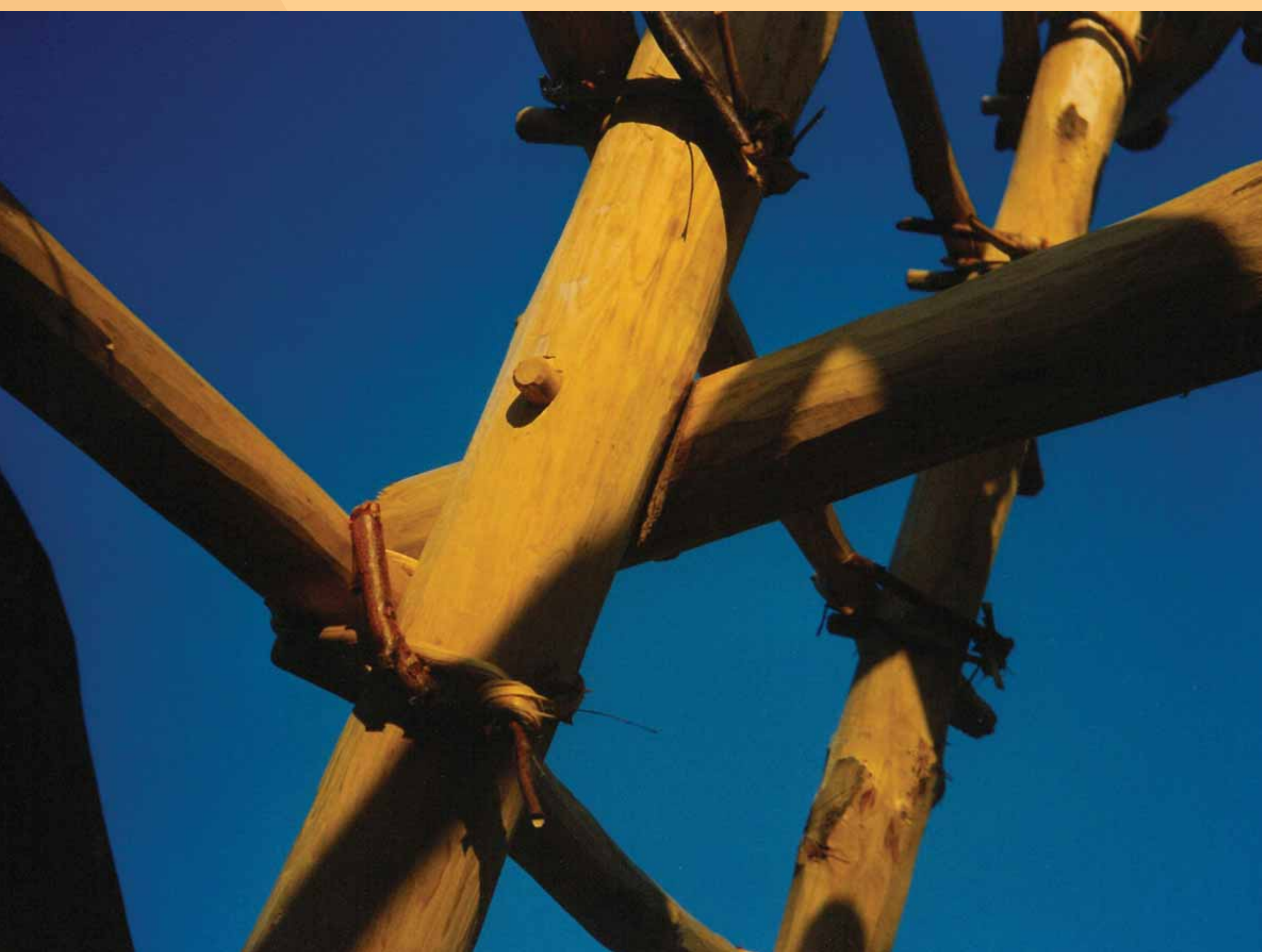
Dettaglio della travatura del tetto
